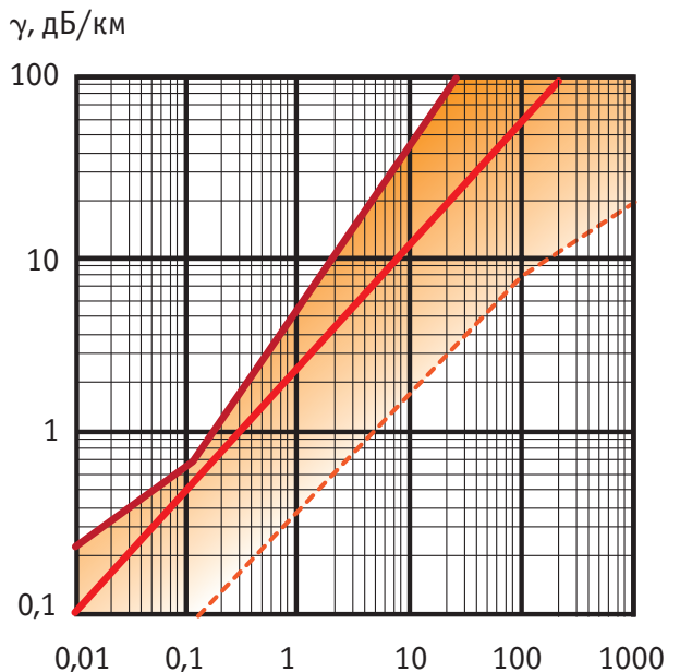
Рис. 1. Ослабление ИК-излучения для различных погодных условий
