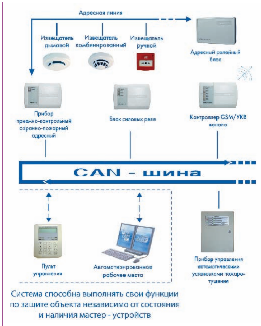
Рис. 2. Система безопасности, построенная на базе CAN-шины
