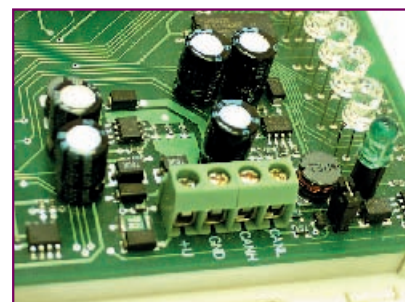
Рис. 1. Плата, поддерживающая CAN
