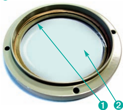
Рис. 8. «Утепление» гермобокса изолятором
