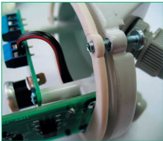
Рис. 7. Передняя крышка гермобокса со стеклом
