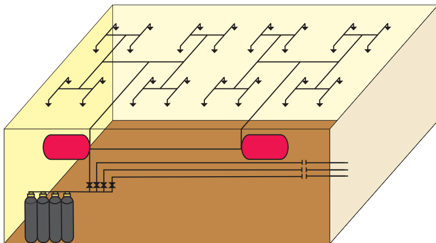
Рис. 1. Помещение большой площади (склад, подземная автостоянка и т.п.)
